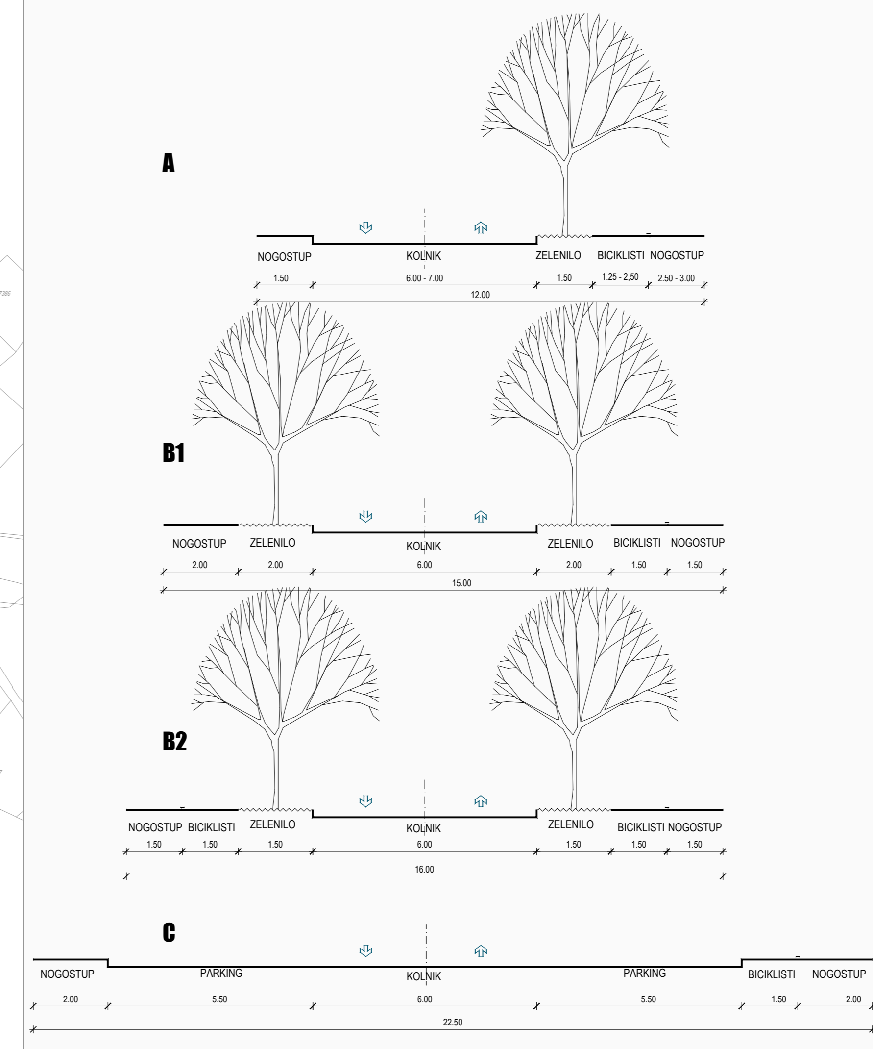
KARAKTERISTIČNI PRESJECI PROMETNICA
